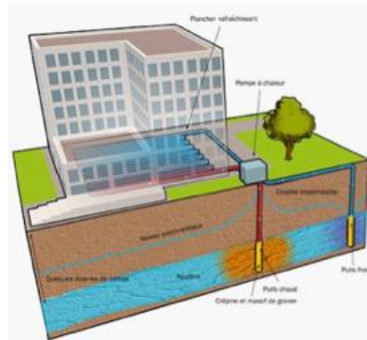
PAC sur aquifère superficiel
